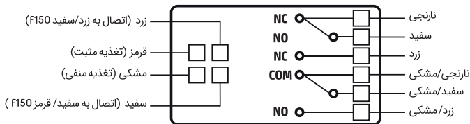
(دیاگرام مازول A100)
